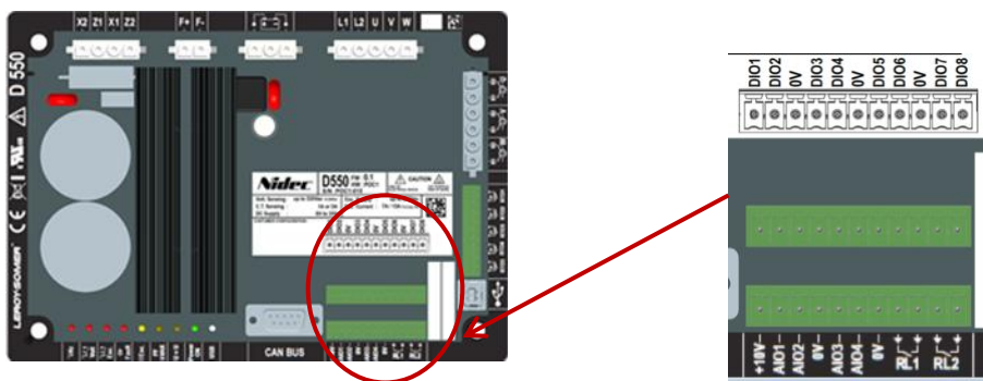
Рисунок 4: Соединение входов/выходов
