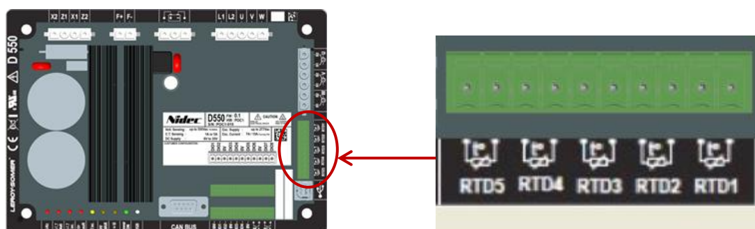
Рисунок 3: Соединения температурного датчика
