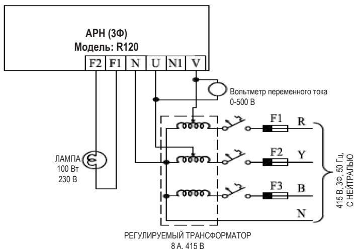
ЭЛЕКТРИЧЕСКАЯ СХЕМА ПРОВЕДЕНИЯ СТАТИЧЕСКИХ ИСПЫТАНИЙ АРН при 3х фазном подключении
