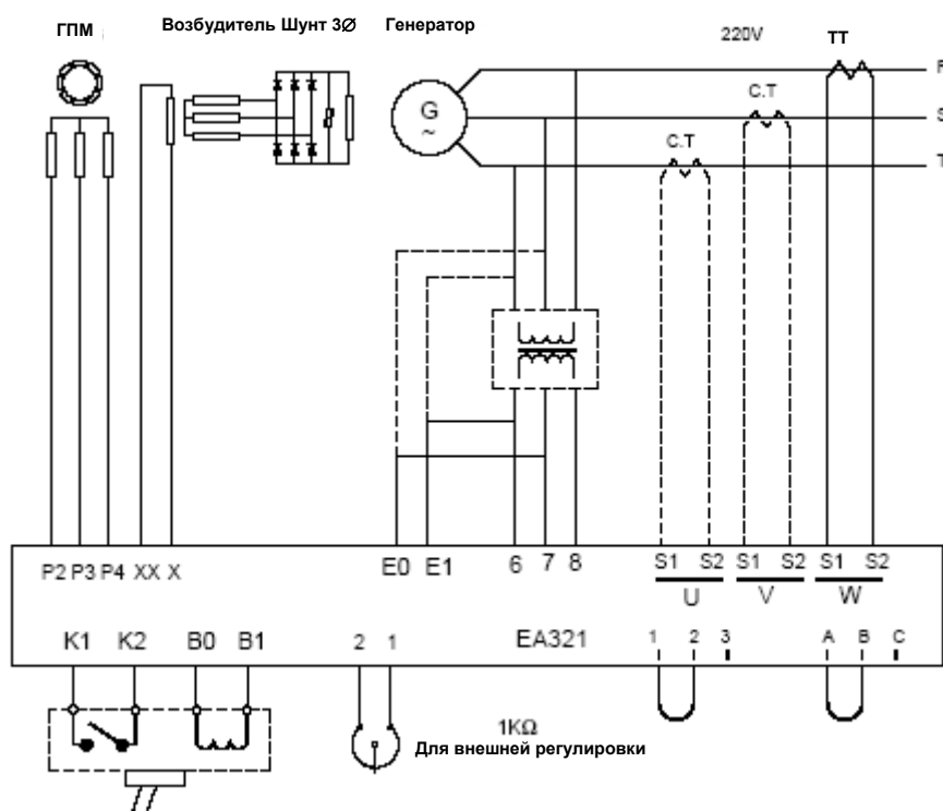
Рисунок 3: Схема разводки
