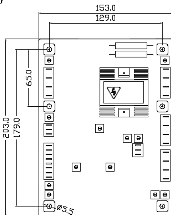
Схематический чертеж Рисунок 1
