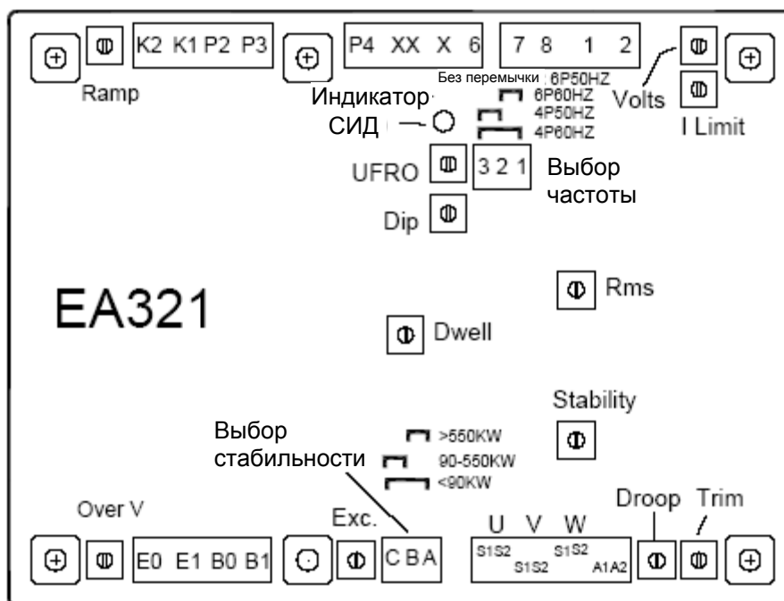
Рисунок 2 Чертеж расположения регуляторов
